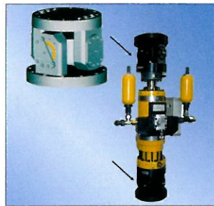
W+B 液压伺服作动器 W+B Servo-hydraulic Actuators
